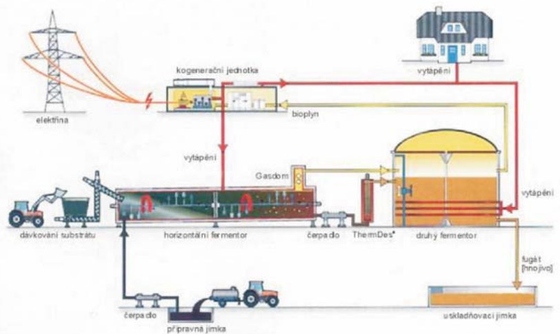
PROCESNÍ SCHÉMA STANDARDNÍ BIOPLYNOVÉ STANICE
